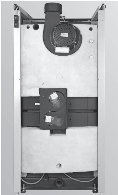
Fig. 63 Monter les isolations de la paroi arrière
