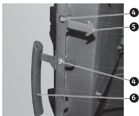
Fig. 18 Monter la poigne et crochet de fermeture avec la vis à téton
