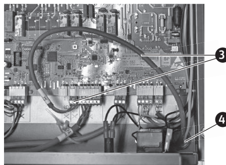
Fig. 70 Faire passer le câble de l'interrupteur de porte et le brancher au connecteur X15
