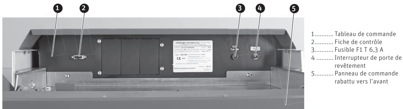
Fig. 84 Tableau de commande chaudière bois à gazéification
