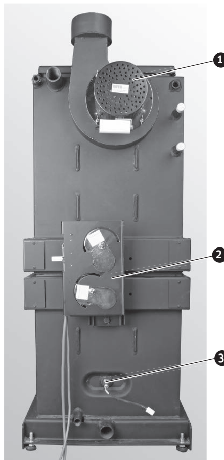
Fig. 32 Ventilateur de fumées, régulation d'air et sonde lambda montés
