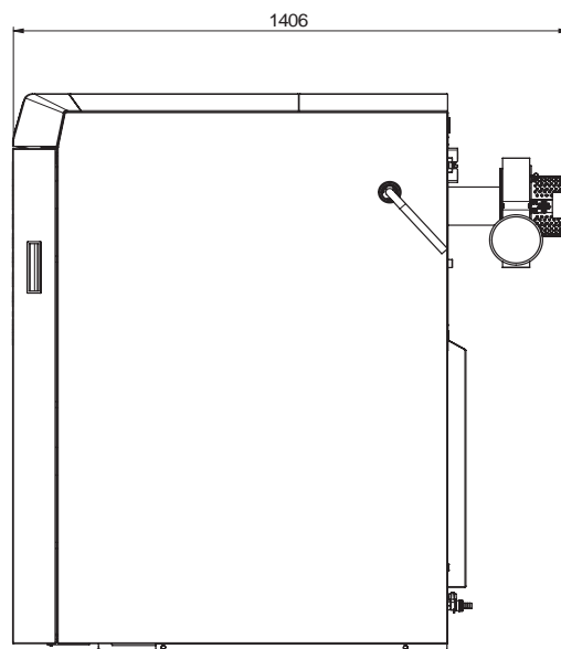
Fig. 97 Ventilateur de fumées monté avec un adaptateur sur la chaudière LogWIN Klassik – Vue du côté droit
