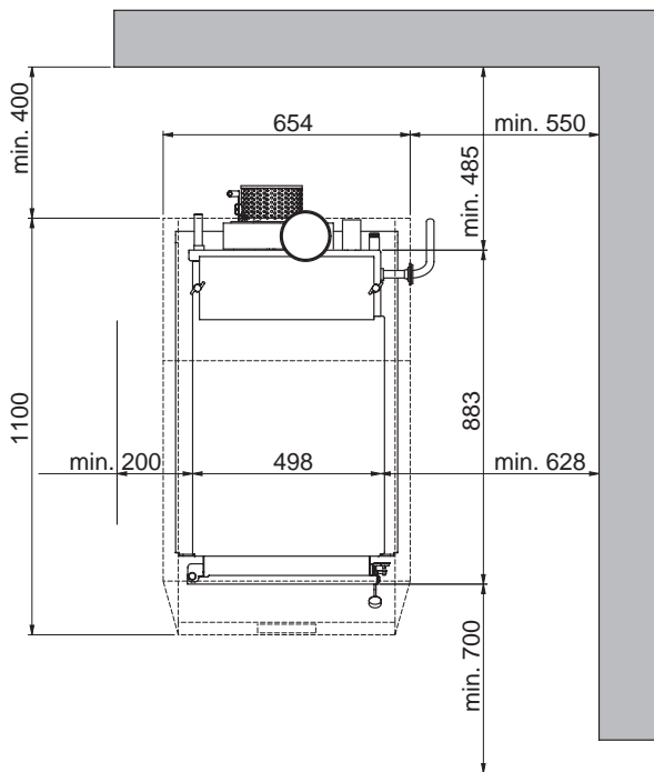
Fig. 5 LogWIN Klassik, tube de fumées vers le haut – Vue du dessus
