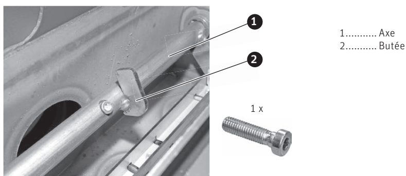
Fig. 41 Visser solidement les arbres ensemble dans l'axe
