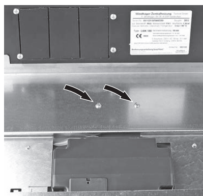
Fig. 77 Régler l'interrupteur de porte à l'aide des vis
