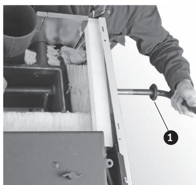
Fig. 67 Dégager l'orifice prédécoupé, engager le levier de nettoyage de la surface d'échange dans l'ouverture
