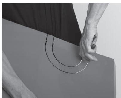
Fig. 80 Lorsque l'adaptateur du raccord d'évacuation des fumées n'est pas utilisé , dégager la partie prédécoupée.
