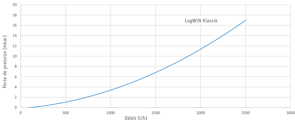
Diagramme 1 Résistance côté eau – LogWIN Klassik
