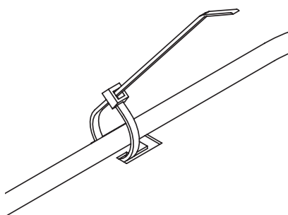
Fig. 90 Fixer les câbles au moyen d'un serre-câbles comme décharge de traction
