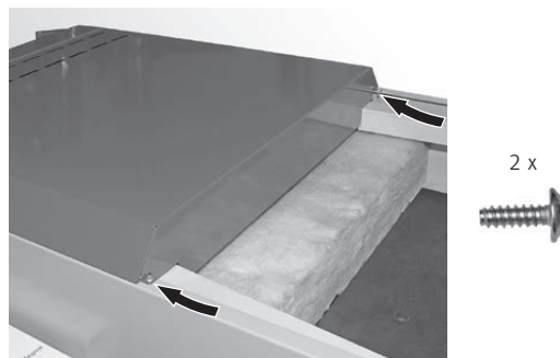
Fig. 79 Fixer le capot de la chaudière à l'aide de 2 vis
