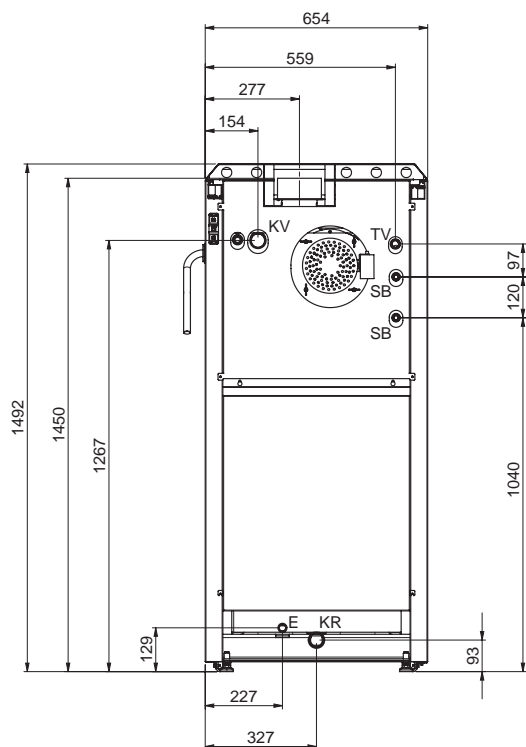
Fig. 94 Ventilateur de fumées monté directement sur la chaudière LogWIN Klassik – vue de la face arrière
