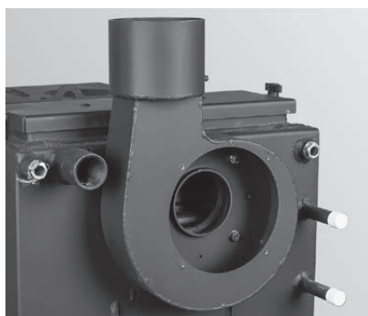
Fig. 10 Volute du ventilateur directement sur la chaudière – configuration de série
