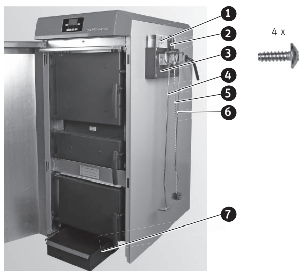
Fig. 82 Monter la console de suspension, tiroir à cendres sous la chaudière
