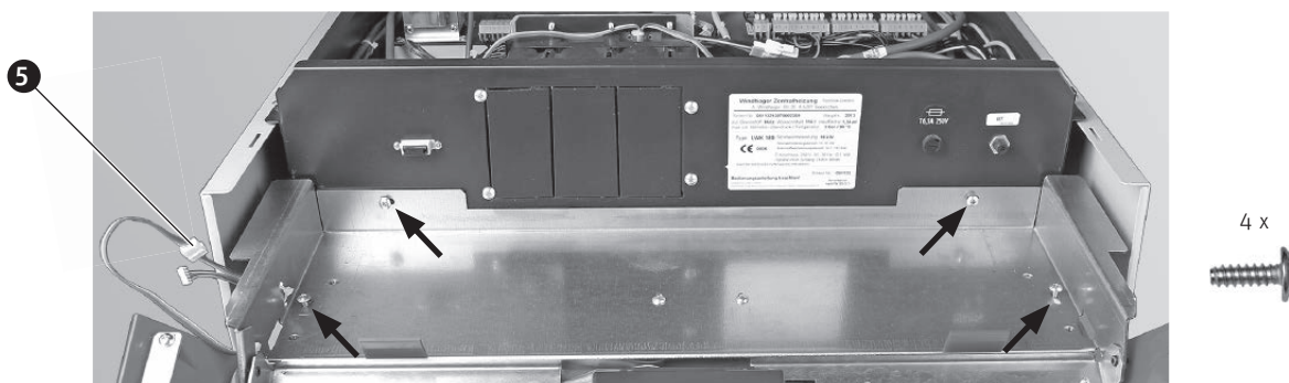
Fig. 71 Fixer le panneau de commande avec 4 vis à tôle, poser le câble InfoWIN PLUS
