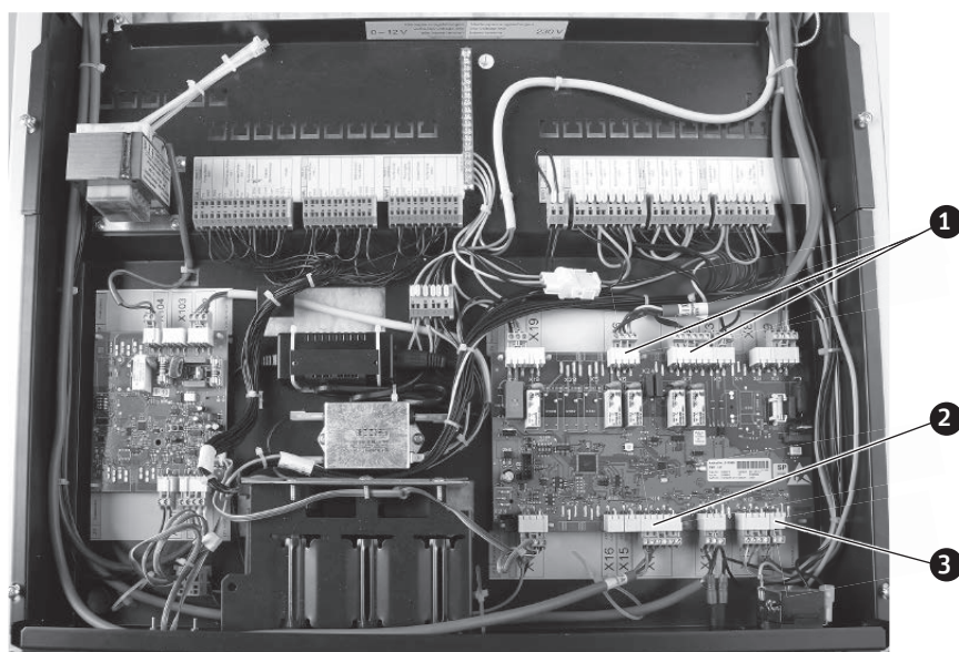
Fig. 62 Tableau de commande – Vue du dessus
