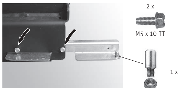
Fig. 9 Monter le gond de la porte de revêtement à gauche ou à droite.
