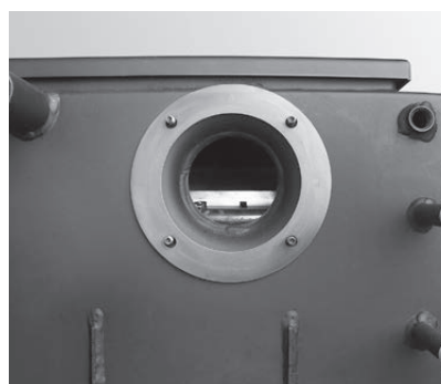
Fig. 13 Joint sur la chaudière
