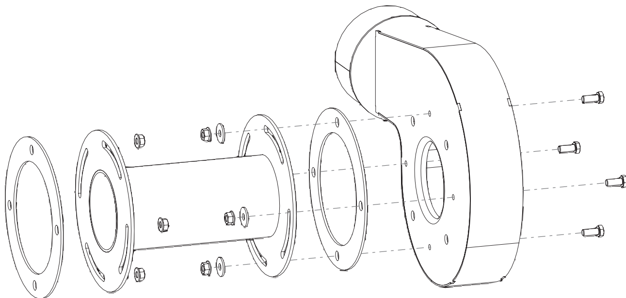
Fig. 66 Monter la volute du ventilateur sur l'adaptateur
