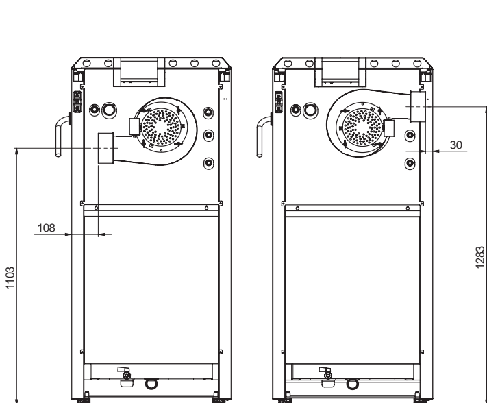
Fig. 96 Ventilateur de fumées monté avec un adaptateur sur la chaudière LogWIN Klassik – vue de la face arrière
