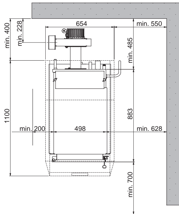
Fig. 6 LogWIN Klassik avec adaptateur pour tube de fumées – Vue du dessus
