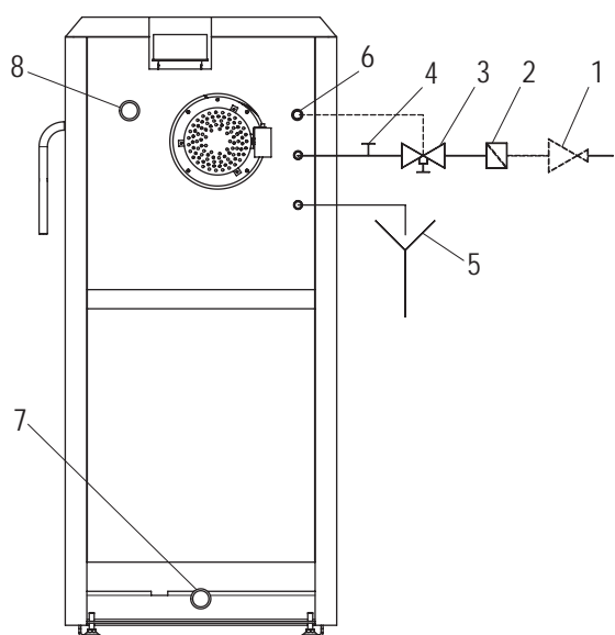
Fig. 83 Raccordement de la batterie de sécurité
