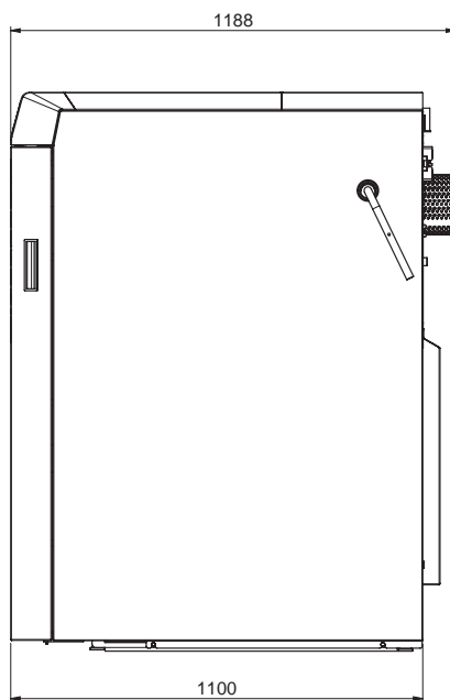
Fig. 95 Ventilateur de fumées monté directement sur la chaudière LogWIN Klassik – vue du côté droit
