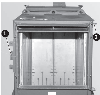
Fig. 16 Intervertir le support de porte et le palier de fermeture
