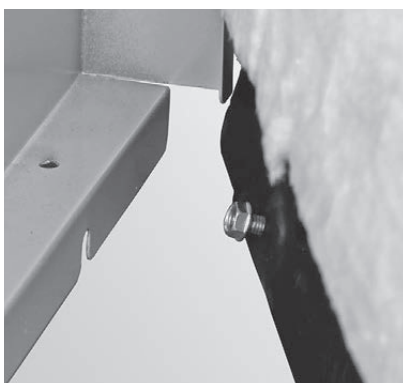
Fig. 49 Accrocher les parois latérales en bas au niveau des vis
