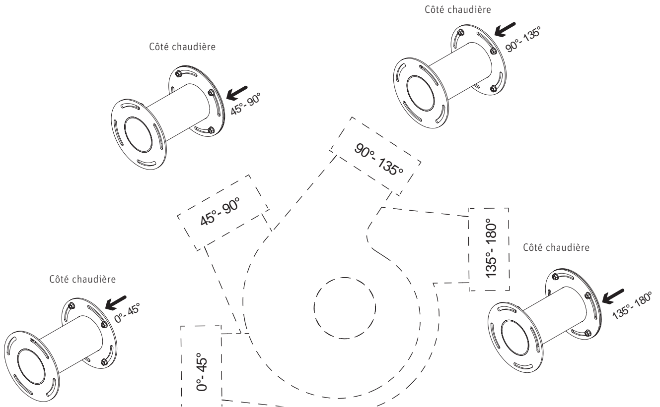
Fig. 14 Montage de l'adaptateur en fonction de l'angle du raccord d'évacuation des fumées
