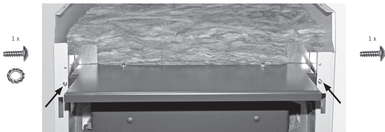
Fig. 51 Visser les parois latérales sans serrer en haut à l'avant
