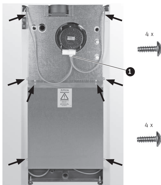
Fig. 65 Monter les parois arrière
