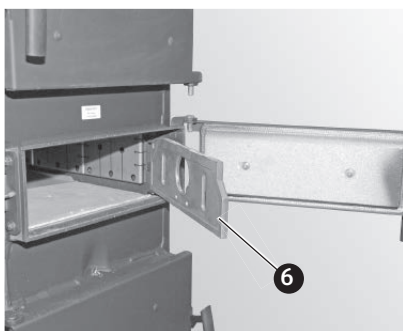
Fig. 24 Porte d'allumage : décrochez la grille verticale et l'accrochez au côté opposé
