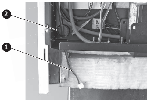
Fig. 69 Faire passer le câble InfoWIN PLUS
