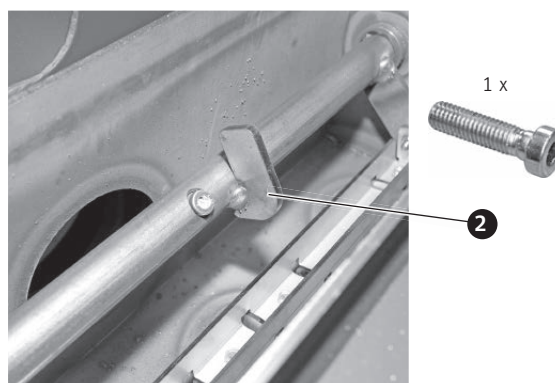
Fig. 68 Enfoncer le levier dans l'axe et le fixer à l'aide d'une vis (seulement engagée)
