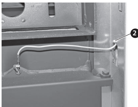
Fig. 57 Tirer le câble en arrière et le fixer à l'aide du serre-câbles 2..... Serre-câbles
