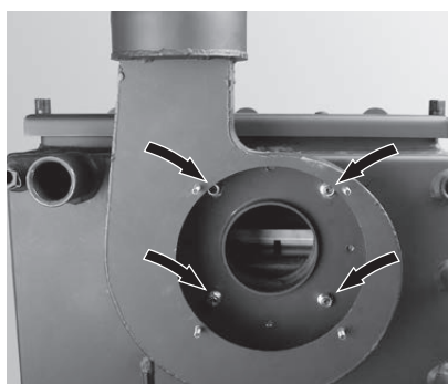
Fig. 12 Dévisser 4 écrous à l'intérieur, au niveau de la volute du ventilateur et retirer la volute
