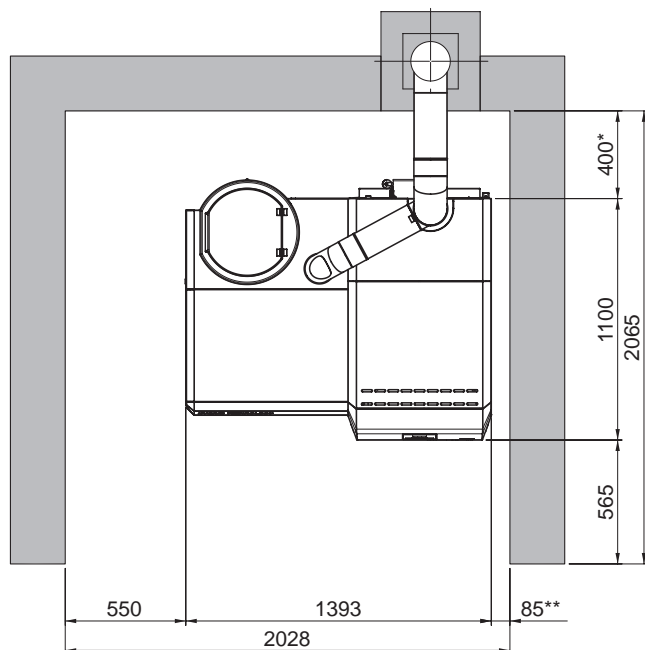
Fig. 7 LogWIN Klassik pellet ready – Vue du dessus
