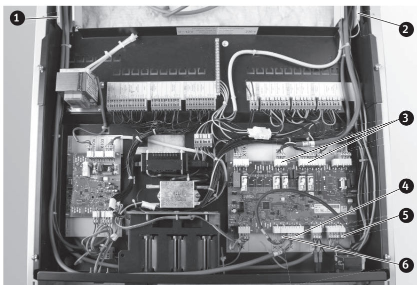
Fig. 89 Ouverture du tableau de commande, branchement des connecteurs – vue avant
