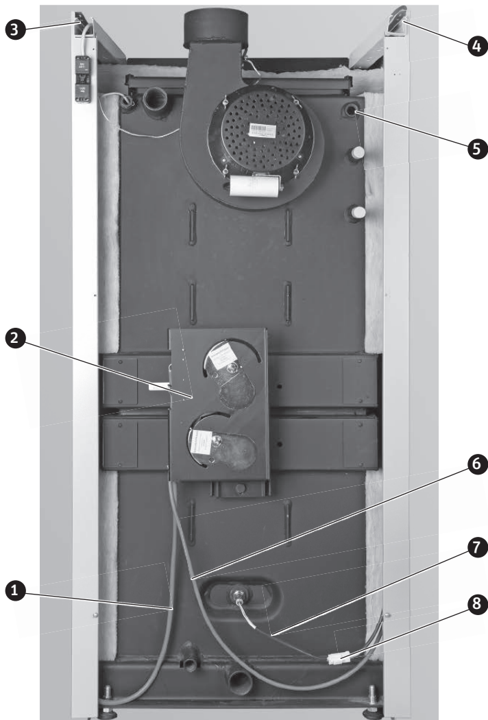
Fig. 61 LogWIN Klassik sans parois arrière – Vue de derrière
