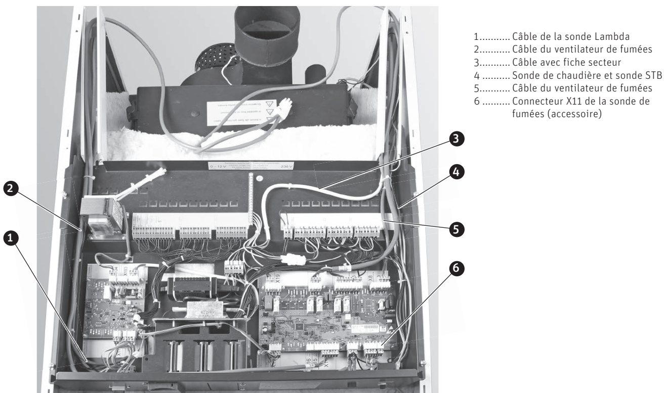
Fig. 59 Tableau de commande, pose des câbles
