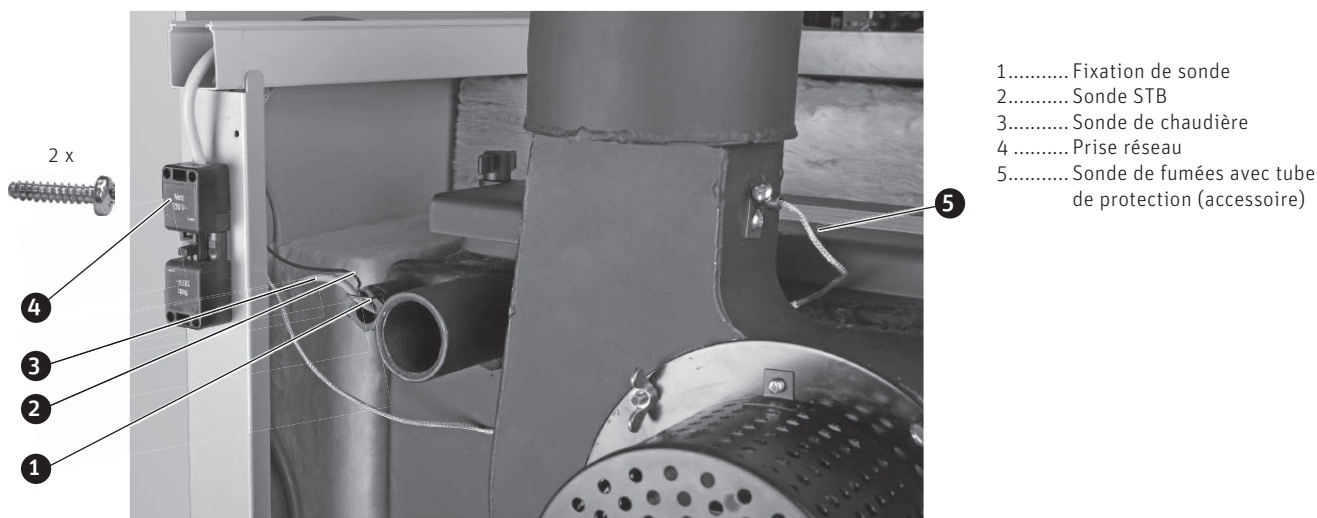
Fig. 60 LogWIN Klassik – Face arrière
