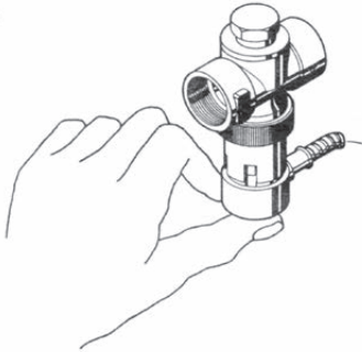
Fig. 93 Sécurité d'écoulement thermique, pression du capuchon rouge contre la soupape
