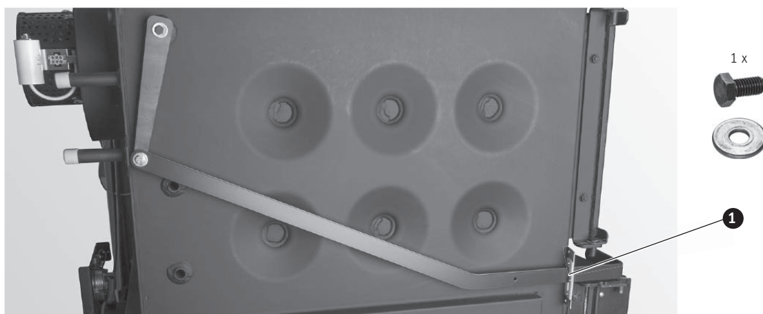
Fig. 40 Visser le levier de nettoyage des surfaces d'échange
