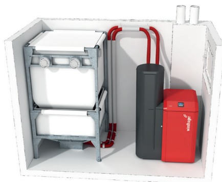
Remplissage automatique
