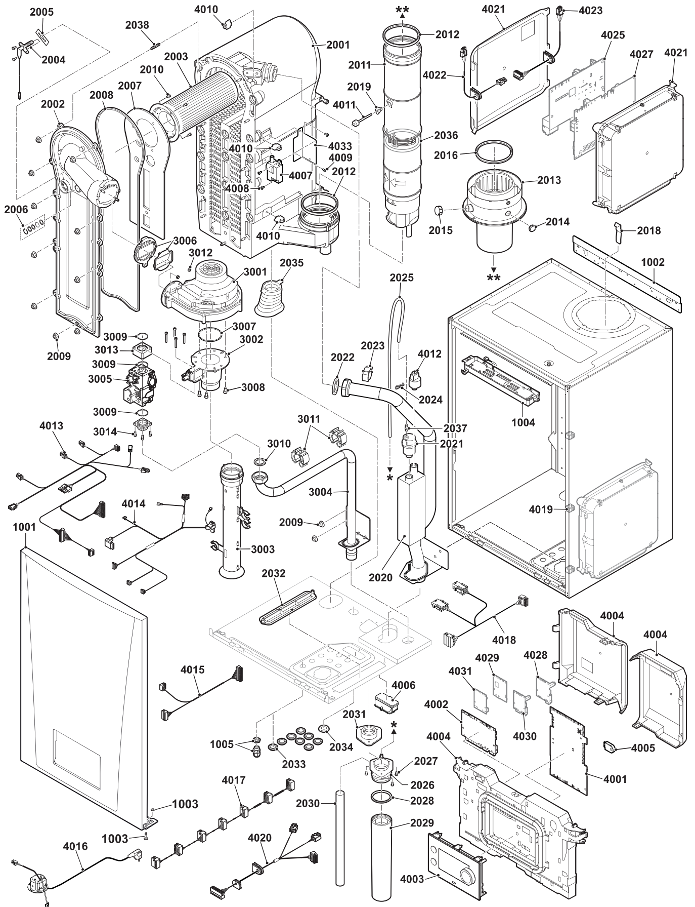
Fig.132 Quinta 115
