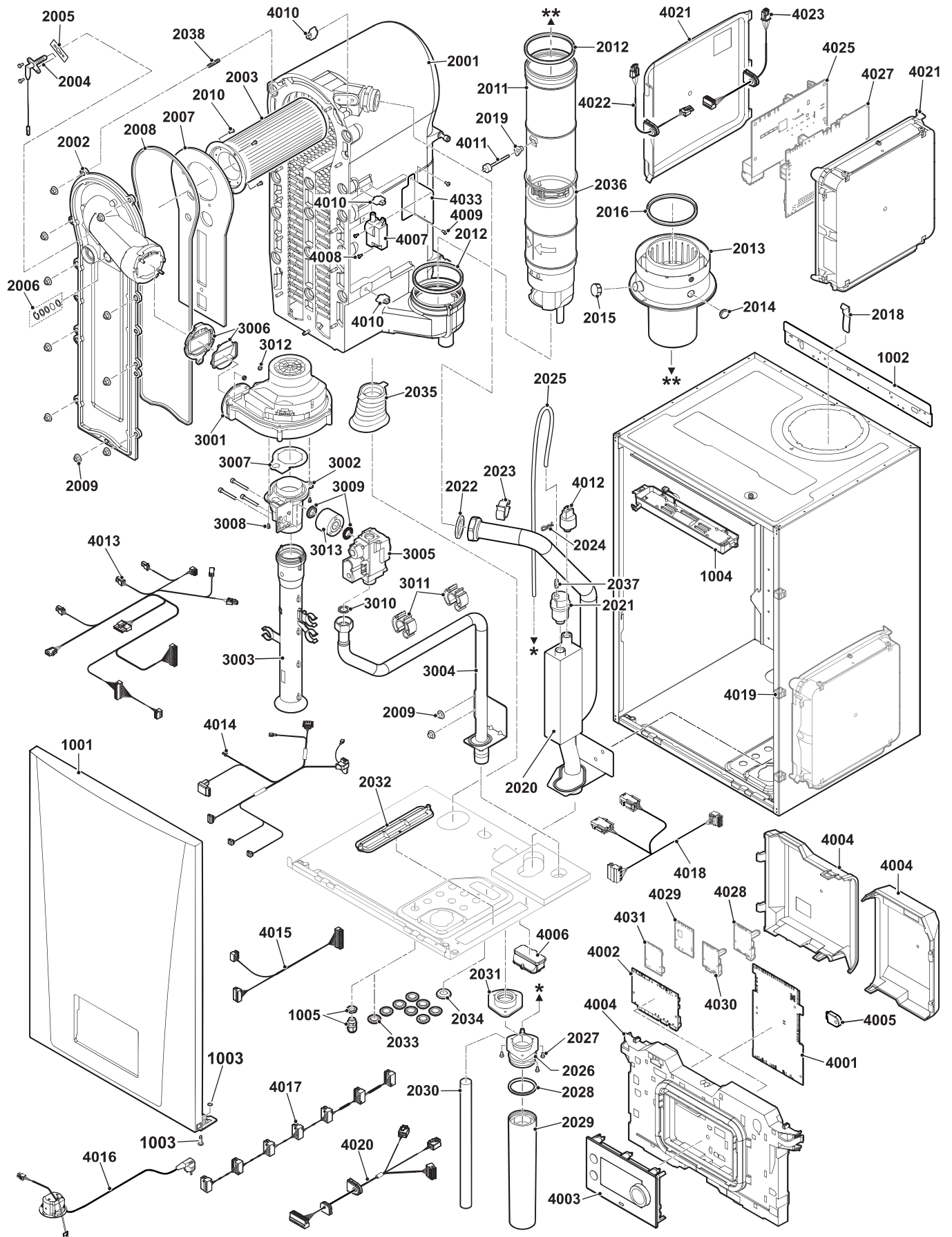
Fig.131 Quinta 90
