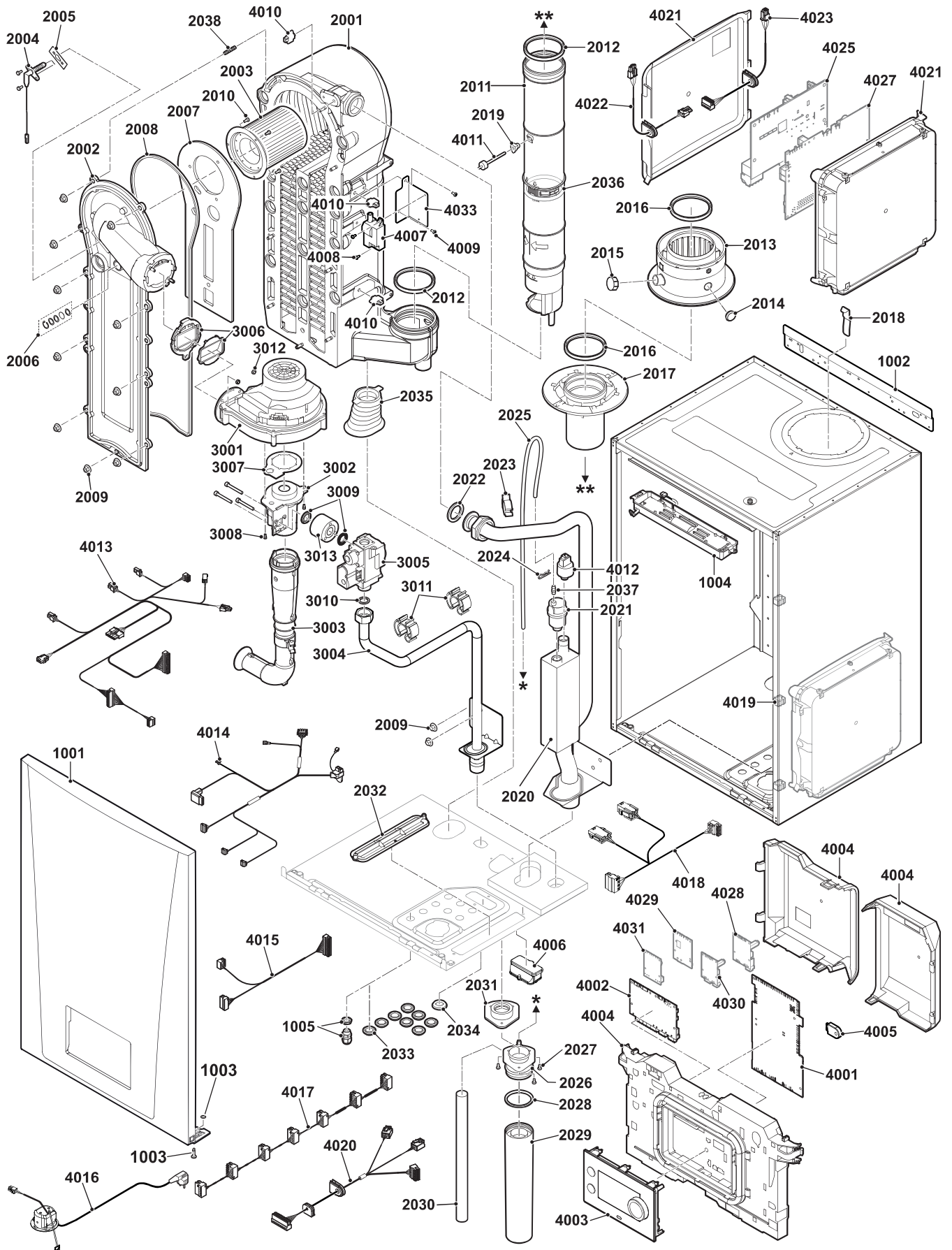
Fig.129 Quinta 45
