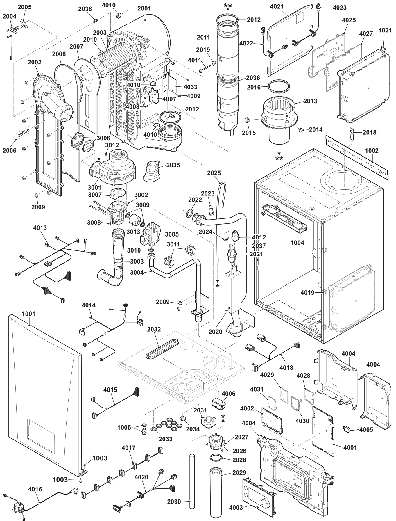
Fig.130 Quinta 65
