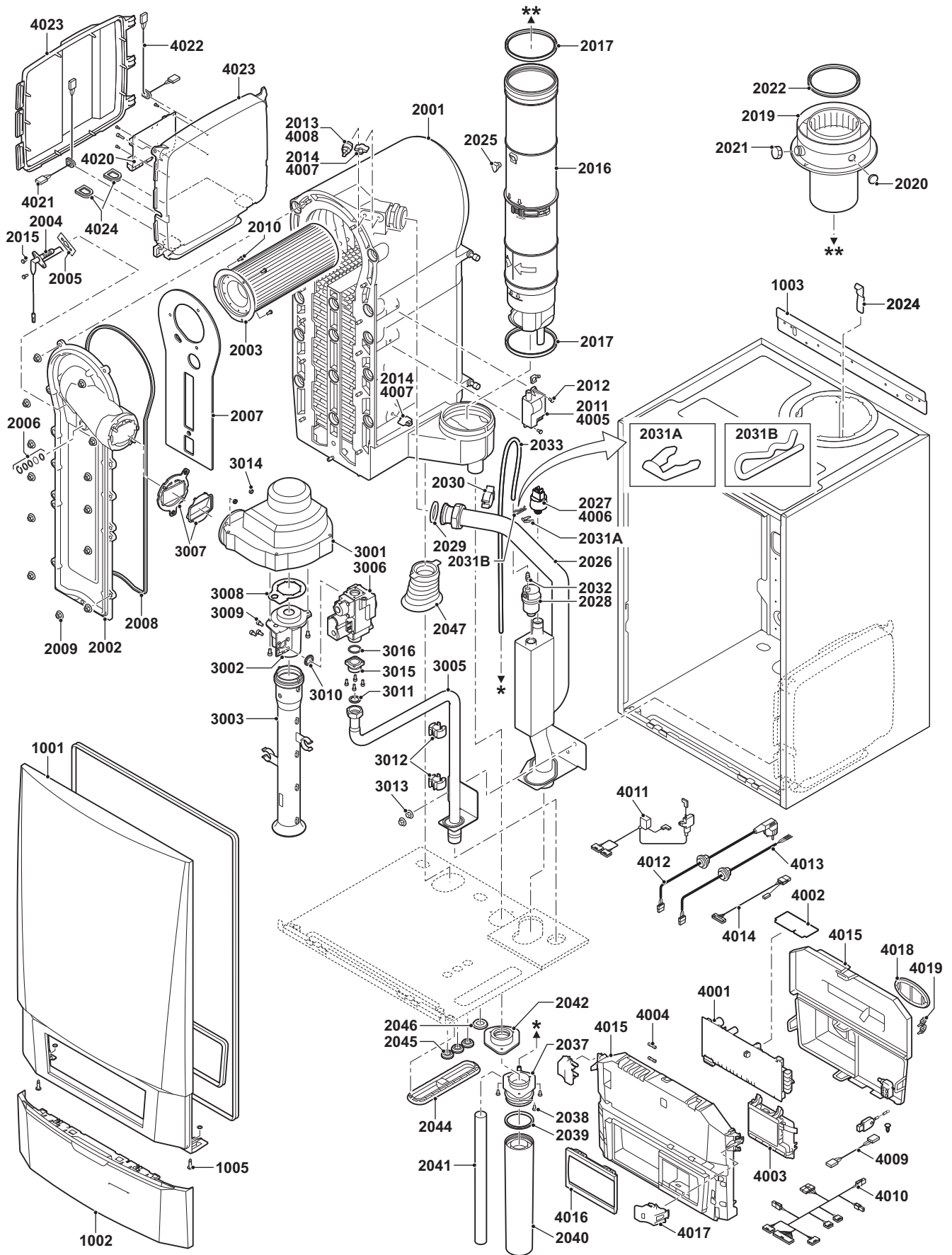
Fig.68 Quinta Pro 90
