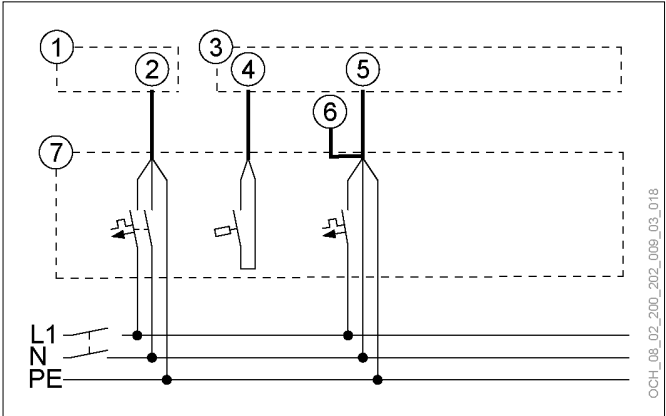
1 Boîtier électrique de l'unité intérieure 2 Distributeur principal de l'installation 3 Alimentation de la pompe à chaleur (compresseur) 4 Contact de signalisation SDE 5 Alimentation du circuit électrique de commande (régulateur OTS) 6 Vanne de retour (normalement fermée) 7 Boîtier électrique de l'unité extérieure
