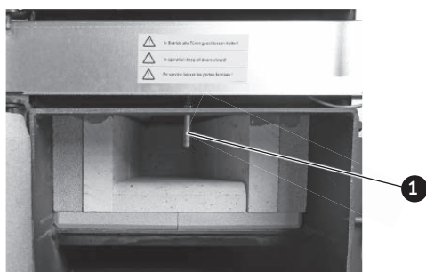
Fig. 40 Nettoyage de la sonde Thermocontrol
