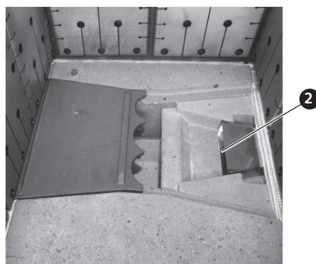
Fig. 42 Sortir les tablettes de combustion, contrôler les ouvertures d'air secondaire.
