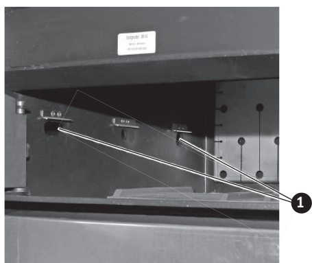
Fig. 41 Décrocher les tôles suspendues ; contrôler les ouvertures d'air primaire.
