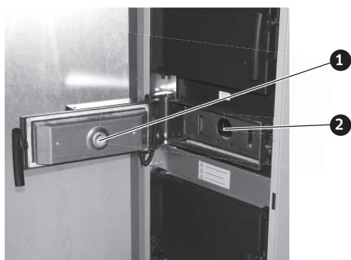
Fig. 30 Contrôler les ouvertures d'allumage
