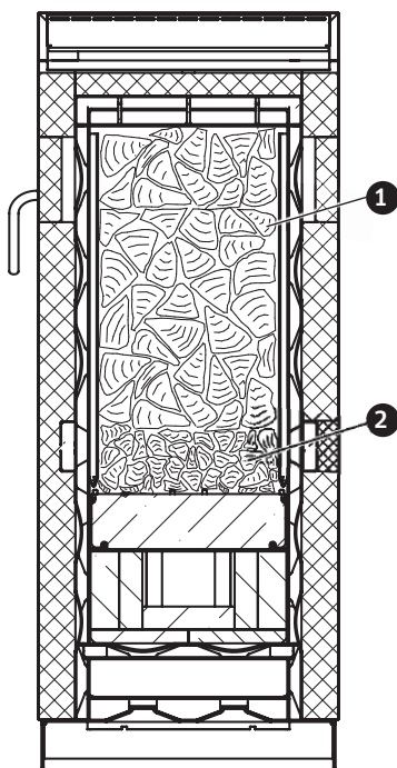
Fig. 12 Vue en coupe du foyer
