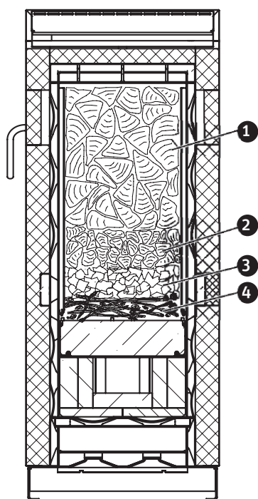
Fig.10 Vue en coupe du foyer
