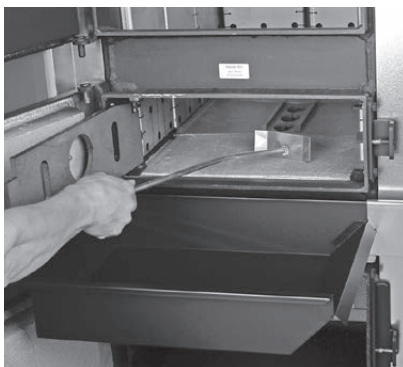
Fig. 8 Accrocher le tiroir à cendres, vider les cendres
