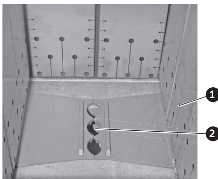
Fig. 9 Foyer, trous des tôles suspendues, ouverture de combustion
