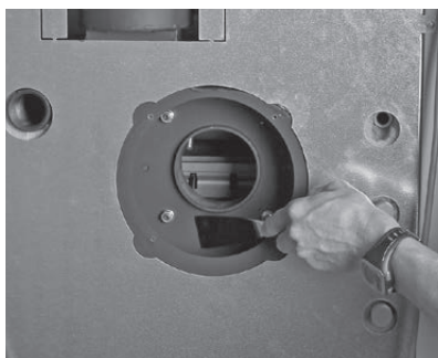
Fig. 37 Nettoyer l'intérieur du caisson de ventilateur
