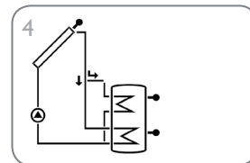
Système de chauffage solaire avec chauffage stratifié du réservoir (page 22)
