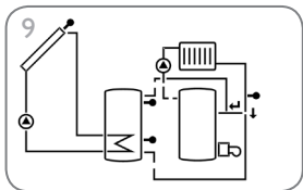
Système de chauffage solaire avec augmentation de la température de retour (page 40)
