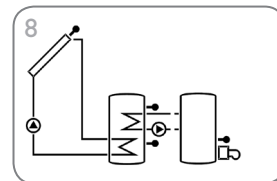
Système de chauffage solaire avec chauffage d'appoint à travers chaudière combustible solide (page 34)
