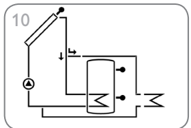
Système de chauffage solaire standard avec évacuation de l'excès de chaleur (page 43)
