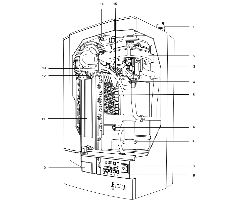
fig. 01 Vue intérieure de la Remeha Quinta 85
