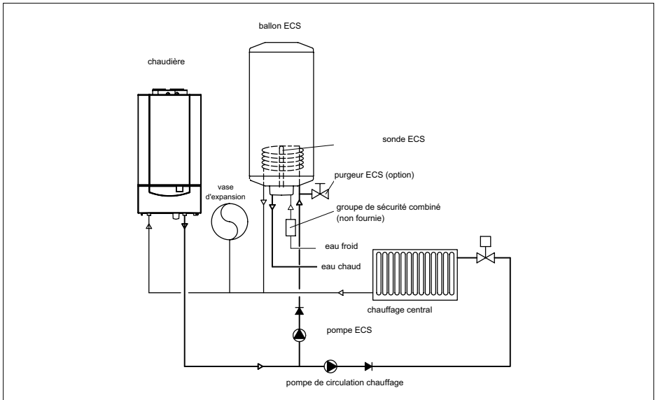
fig. 12 Raccordement d'un ballon ECS à l'aide d'une pompe de charge (schéma de principe)
