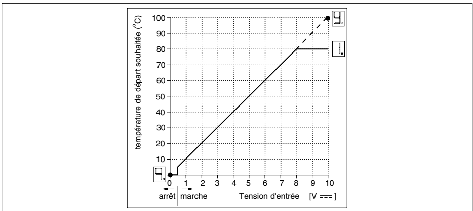
fig. 19 Graphique tension - température
