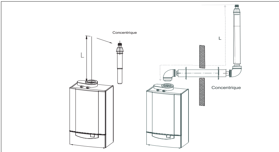
fig. 10 Exécution en ventouse
