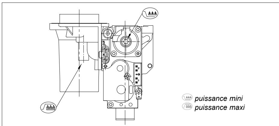
fig. 23 Vis de réglage
