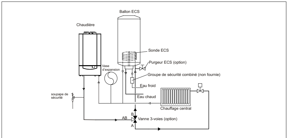
fig. 16 Raccordement avec vanne 3-voies externe
