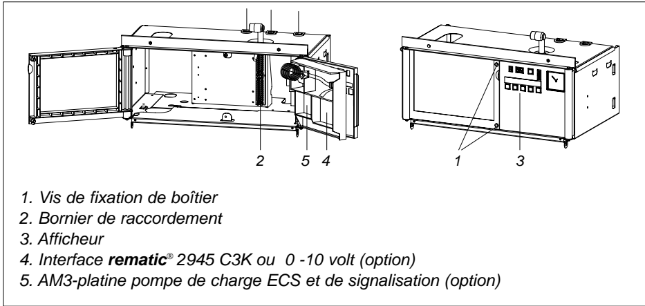
fig. 19 Tableau de bord, vues interne et externe. 00.W3H.79.00054
