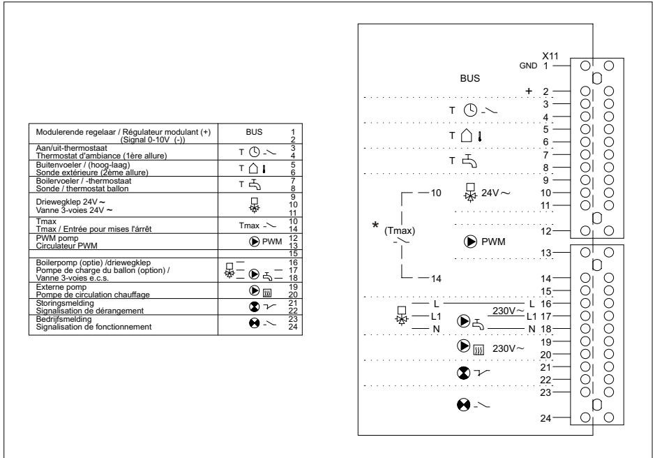
fig. 18 Bornier de raccordement
