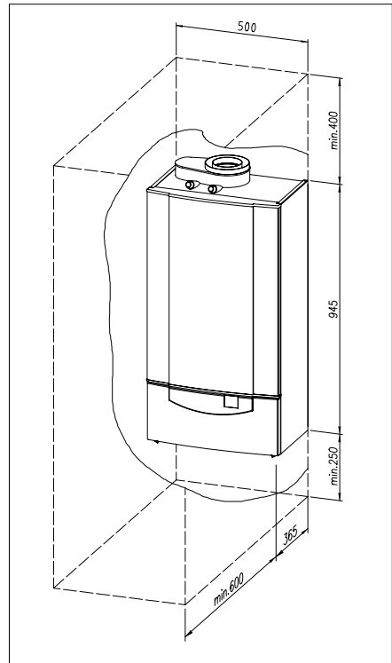
fig. 07 Espace libre Remeha Quinta 05.W3H.79.00065
