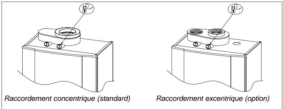
fig. 08 Vue du dessus Remeha Quinta 05.W4H.79.00066 + 00.W3H.79.00049
