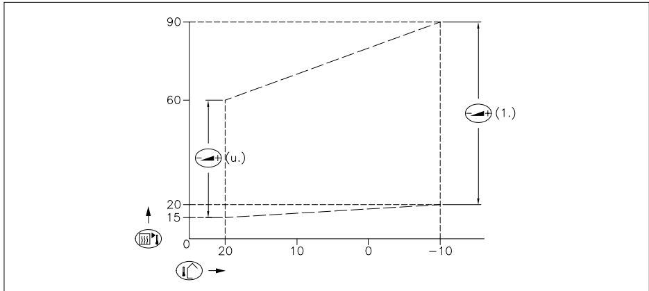
fig. 23 Pente de chauffe interne 00.W4H.79.00017
