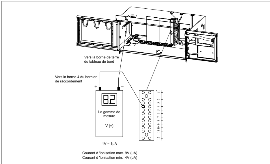
fig. 26 Mesure d'ionisation 06.W3H.79.00002
