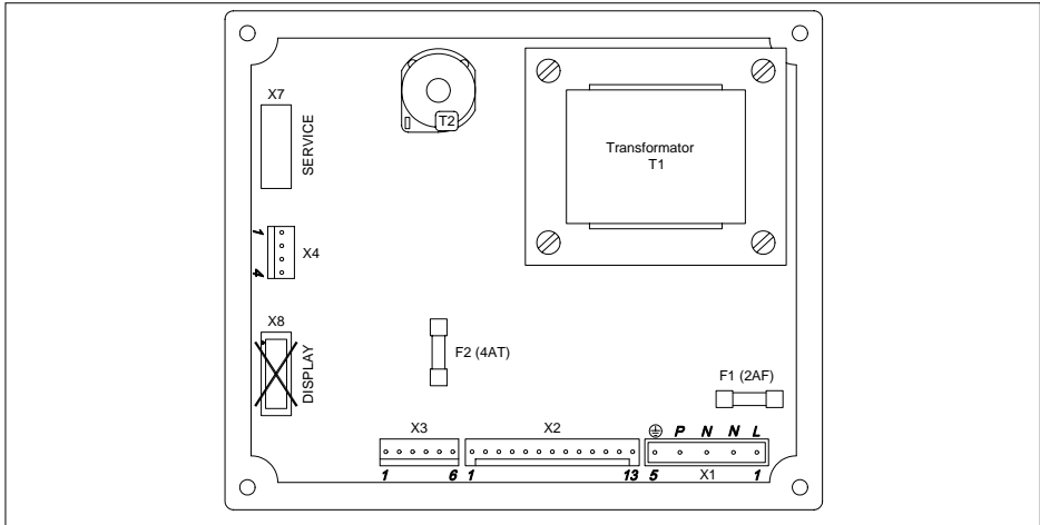
fig. 17 Automate de commande Gasmodul et fusibles 00.W4H.79.00018
