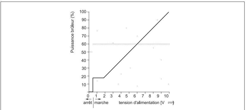
fig. 22 Graphique tension - charge
