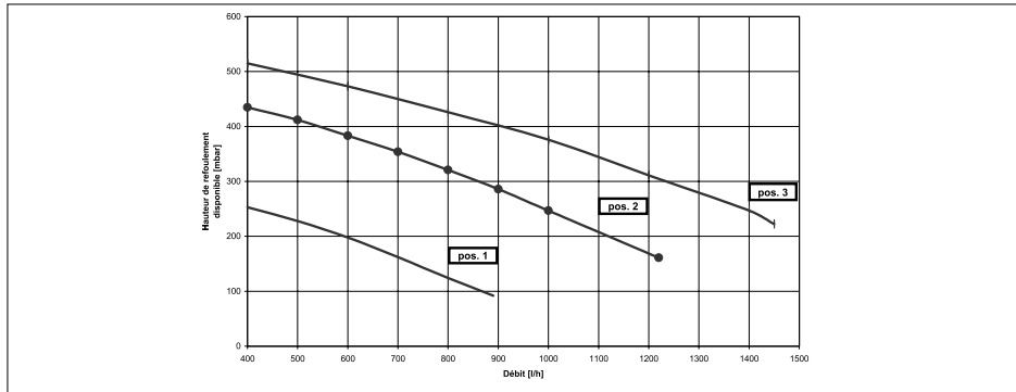
fig. 14 Hauteur de refoulement disponible (Quinta 25s)
