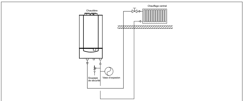
fig. 13 Soupape de sécurité Remeha Quinta 28c et Quinta 35c
