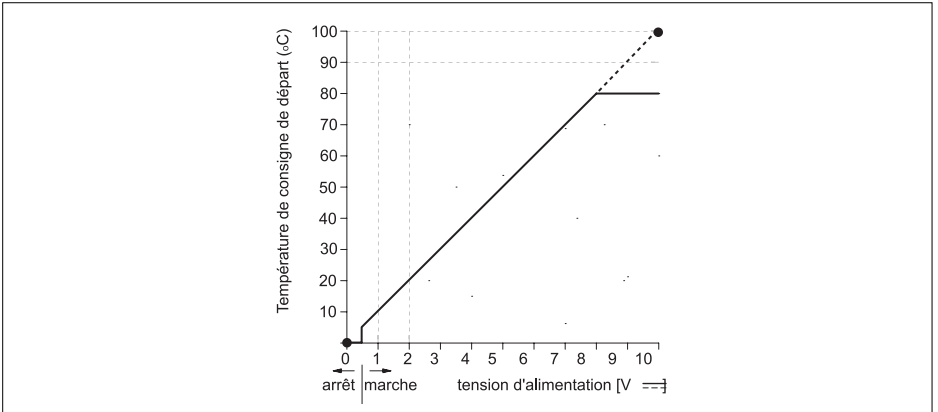
fig. 21 Graphique tension - température
