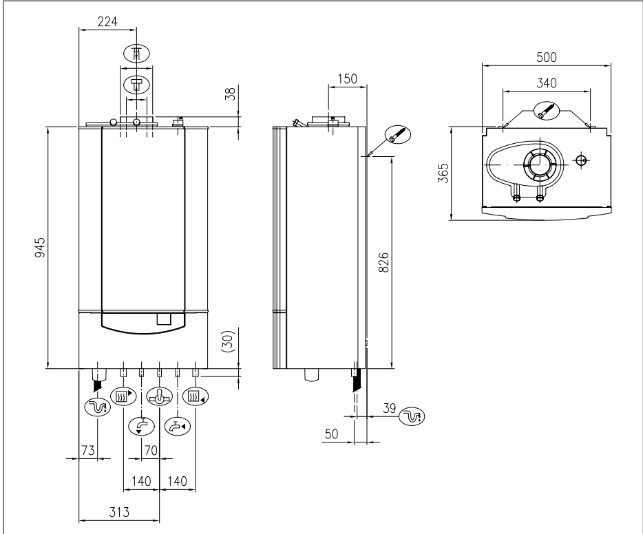
fig. 03 Dimensions Remeha Quinta 28c et 35c
