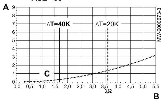
Fig.3 Pertes de charge pour Gas 120 ACE - 115
