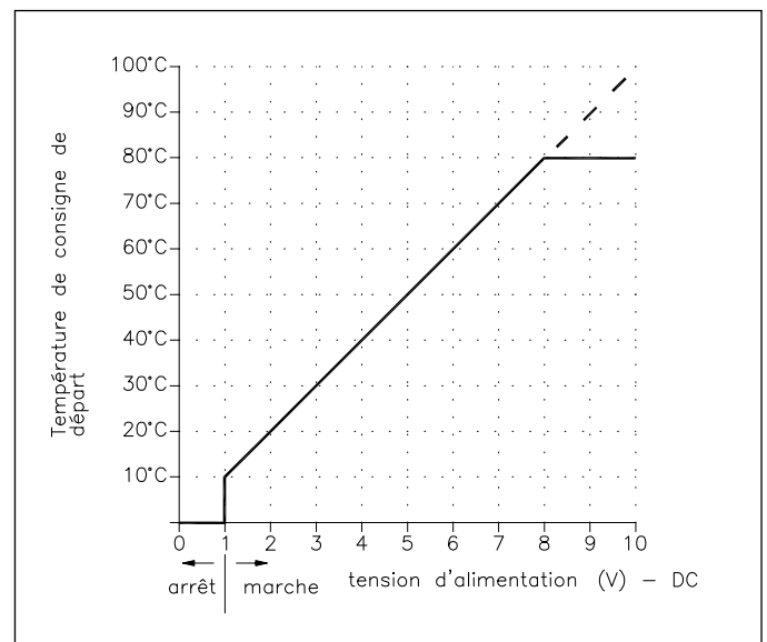
fig. 18 Régulation de la température via le signal analogique (0-10V)
