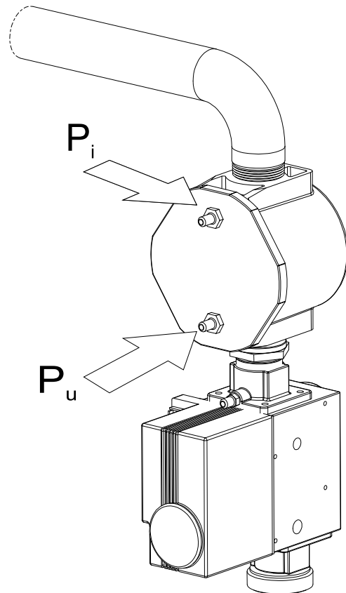
fig. 26 filtre à gaz avec points de mesure
