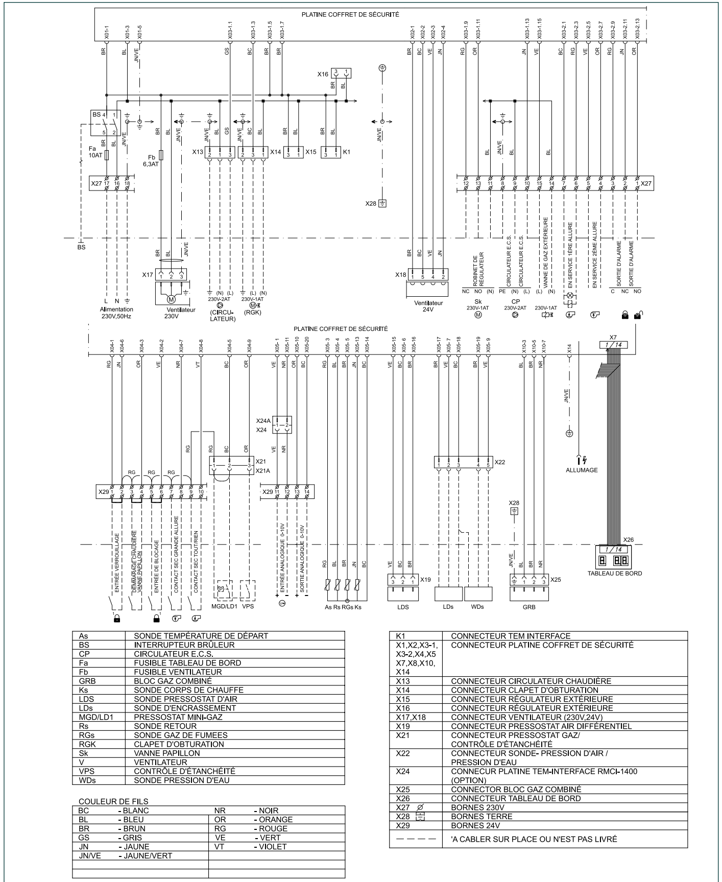
fig. 15 Schéma électrique
