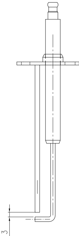
fig. 25 électrode d'allumage
