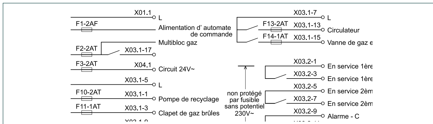
fig. 13 Plan des fusibles
