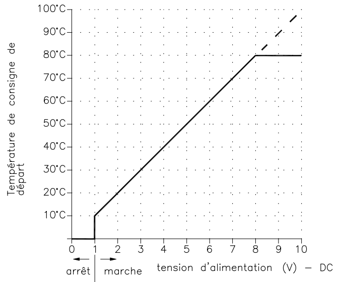
fig. 24 Réglage du signal analogique
