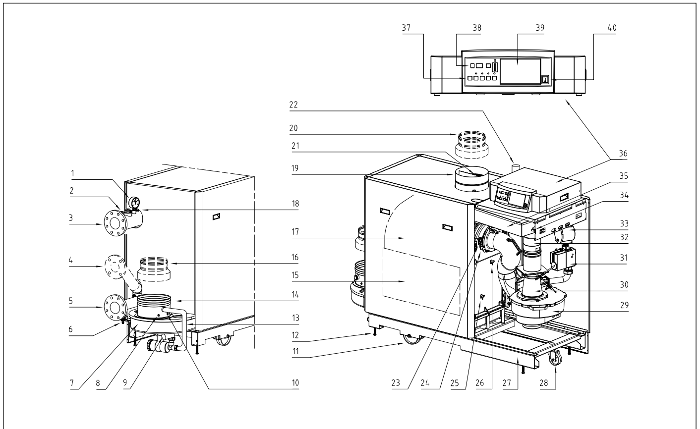
fig. 02 Vue intérieure de la Remeha Gas 310 ECO
