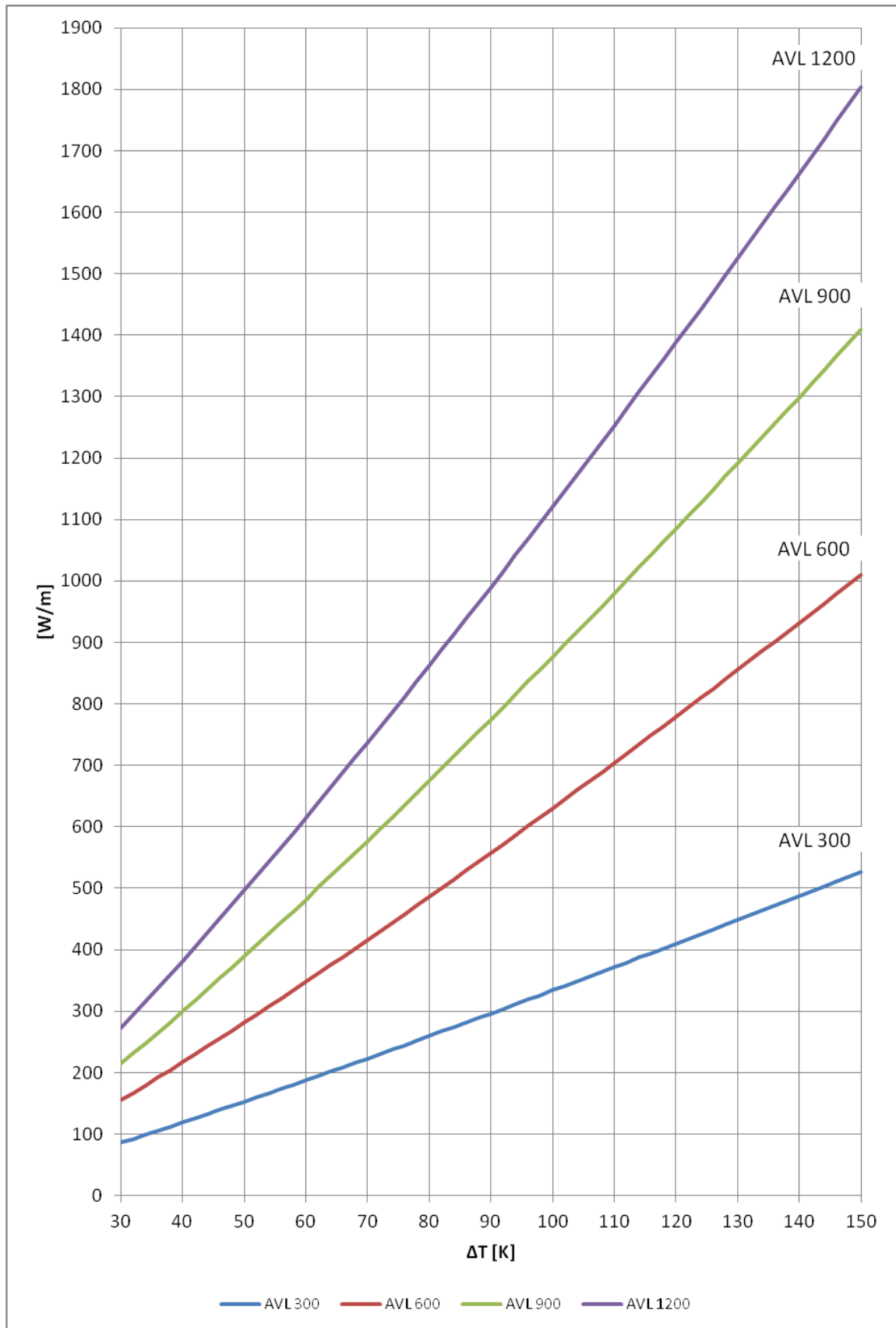
Fig. 1.20 Thermal output for EUTERM AVL
