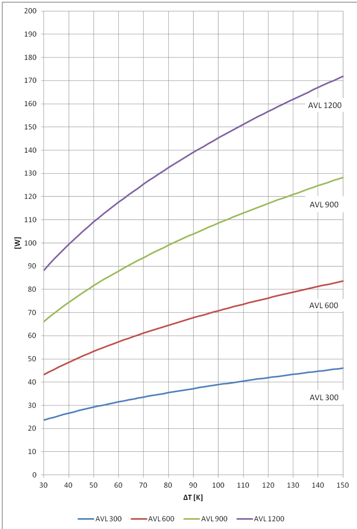
Fig. 1.21 Thermal output for EUTERM AVL headers
