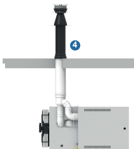
Kit ventouse toiture C32
